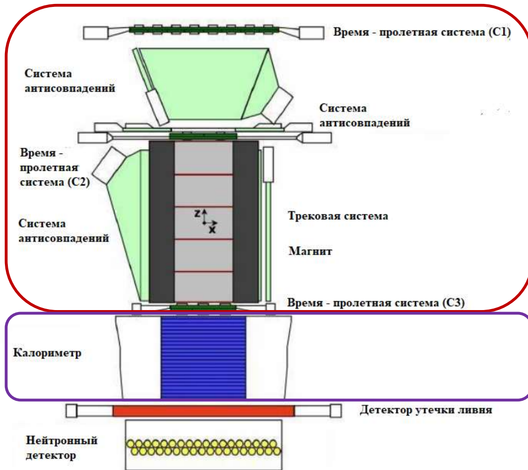
Схема научной аппаратуры PAMELA
