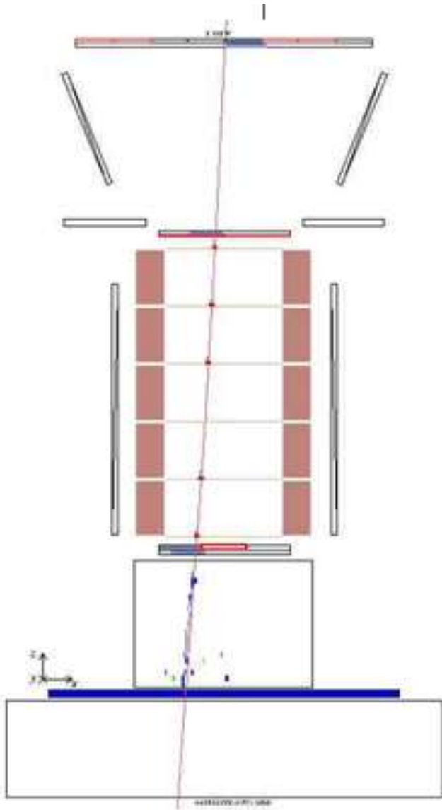
Визуализация взаимодействующего в калориметре события
